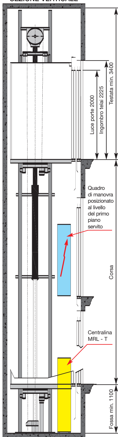
SEZIONE VERTICALE
