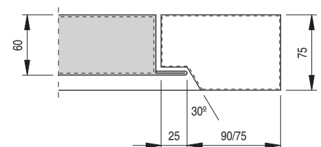
DETALLE E; E. 1/5 DETAIL E; E. 1/5
