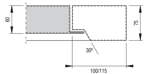
DETALLE E; E. 1/5 DETAIL E; E. 1/5
